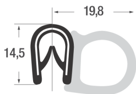
Flexibles Kantenschutzdichtprofil Kantenschutz PVC mit eingebettetem Stahlklemmband und oben aufgesiegelt Moosgummi Dichtschlauch EPDM Klemmbereich 1.0 bis 4.0 mm
