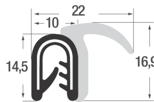
Flexibles Kantenschutzdichtprofil Kantenschutz PVC mit eingebettetem Stahlklemmband und oben aufgesiegelt Moosgummi Dichtschlauch EPDM Klemmbereich 1.0 bis 4.0 mm
